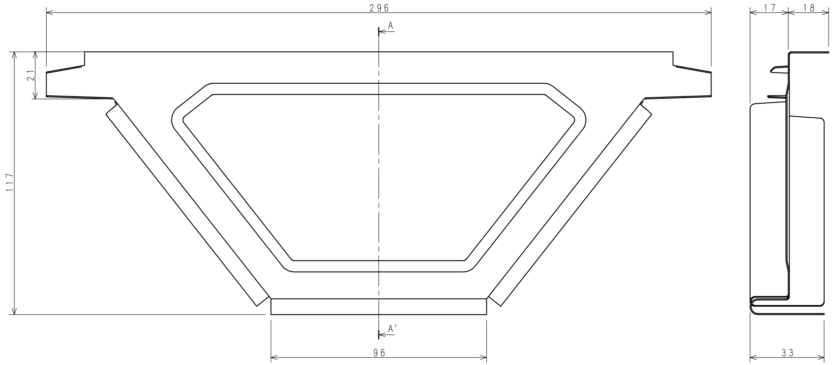
A-A' 断面
